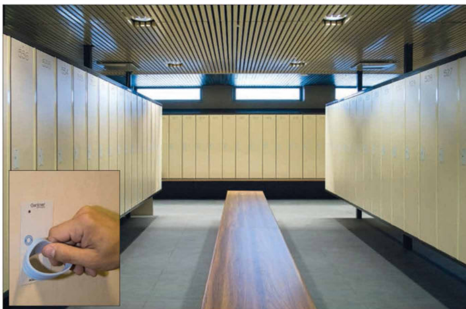
PUNTA VKP skabe med et understel med svævende udtryk. Dørene er udført i kompaktlaminat med indgraveret nummer. Gantner EL lås er tilkoppet svømmehallens elektroniske overvågningssystem. Dørene åbnes med et armbånd. Alle skabe kan kontrolleres fra en PC i receptionen. Låsen har sensor der alarmer ved indbrud.
